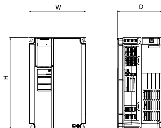
FRN0039LM2A-4E - FRN0045LM2A-4E
