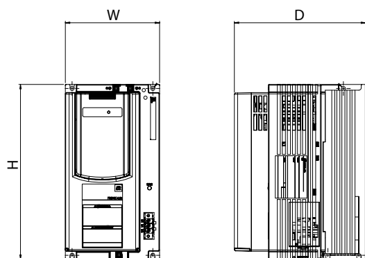
FRN0039LM2A-4E - FRN0045LM2A-4E
